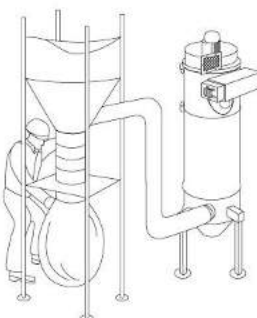
装袋作业 Bagging
