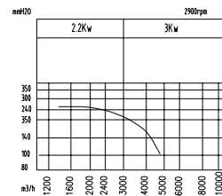
风机风量风压曲线图
