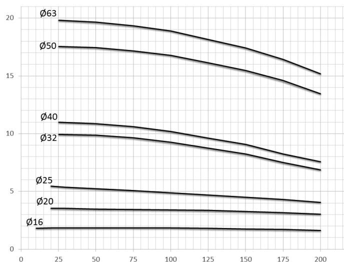
Максимально допустимый момент (M1) как функция хода
