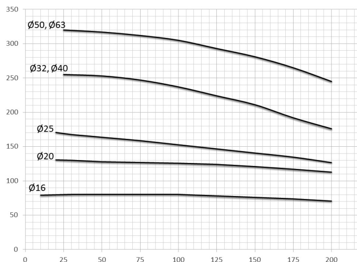
Максимально допустимая нагрузка (F1) как функция хода
