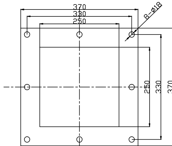
上下对接法兰
